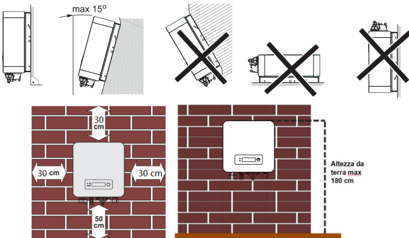
Figura 9 - Requisiti di installazione per un singolo inverter
