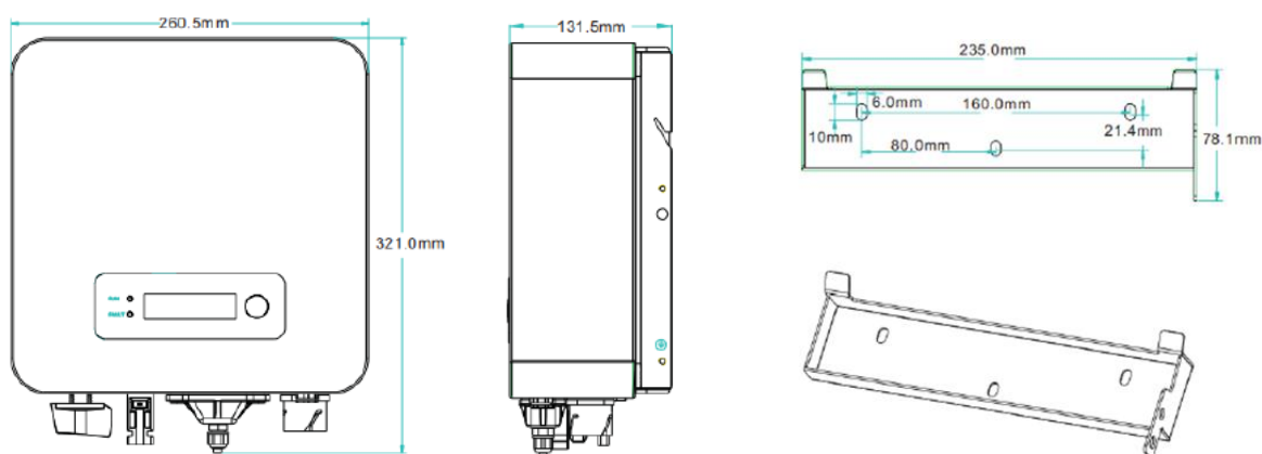
Figura 4 - Vista frontale, laterale e posteriore dell'inverter e della staffa
