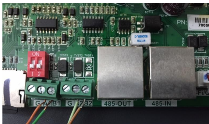
Figura 81 – Collegamento della linea seriale tramite la morsettiere RS485 e la presa RJ45
