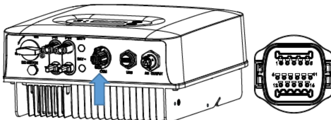
Figura 23 - Vista dal basso dell'inverter 1PH 3000TLM-6000TLM-V3
