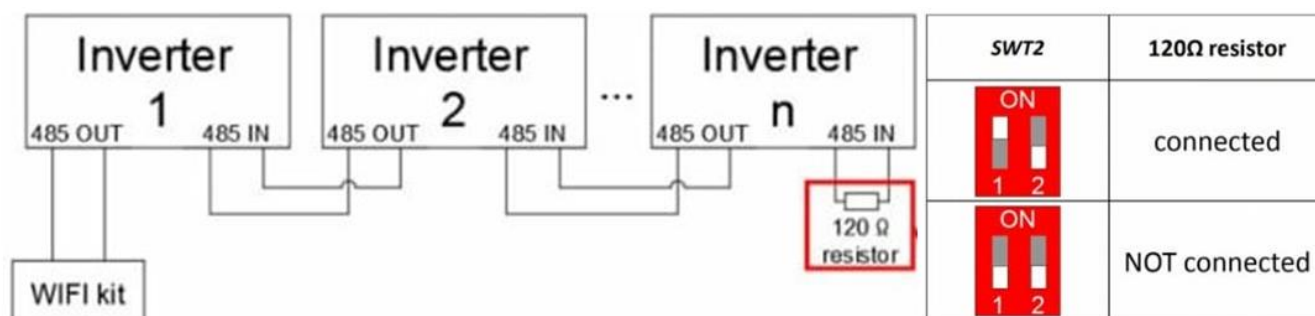
Figura 83 – Posizionamento dei dip switch per il collegamento della resistenza di isolamento
