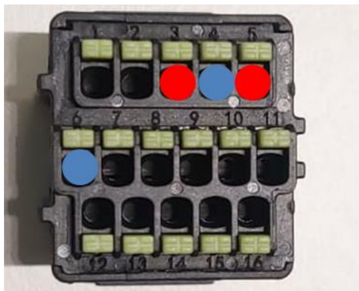
Figura 82c – Collegamento della linea seriale tramite connettore di comunicazione per 3PH HYD5000-HYD20000-ZSS
