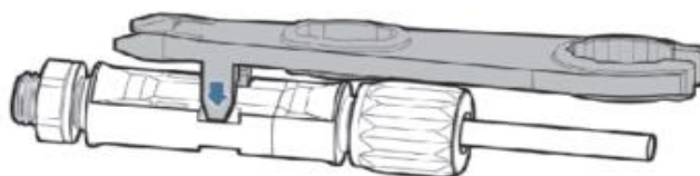
Figura 16 – Rimozione del connettore CC
