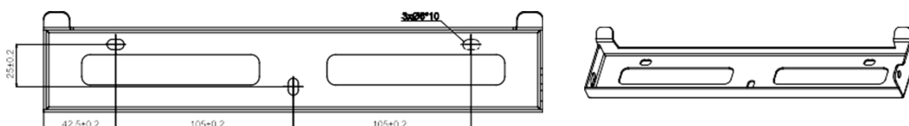
Figura 4 - Dimensioni della staffa
