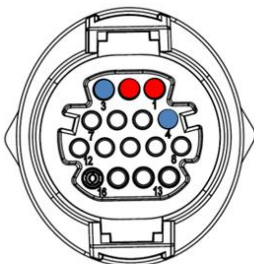
Figura 82a – Collegamento della linea seriale tramite connettore di comunicazione per 3PH HYD5000-HYD20000-ZSS
