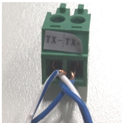
Figura 80 – Serraggio del cavo di rete alla morsettiere RS485
