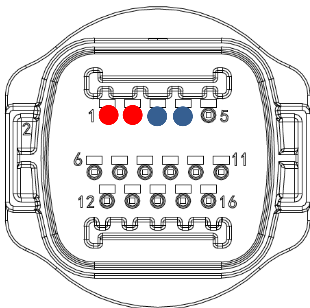
Figura 82b – Collegamento della linea seriale tramite connettore di comunicazione per 1PH 3000-6000 TLM-V3 e HYD 3PH 5000-20000 ZSS
